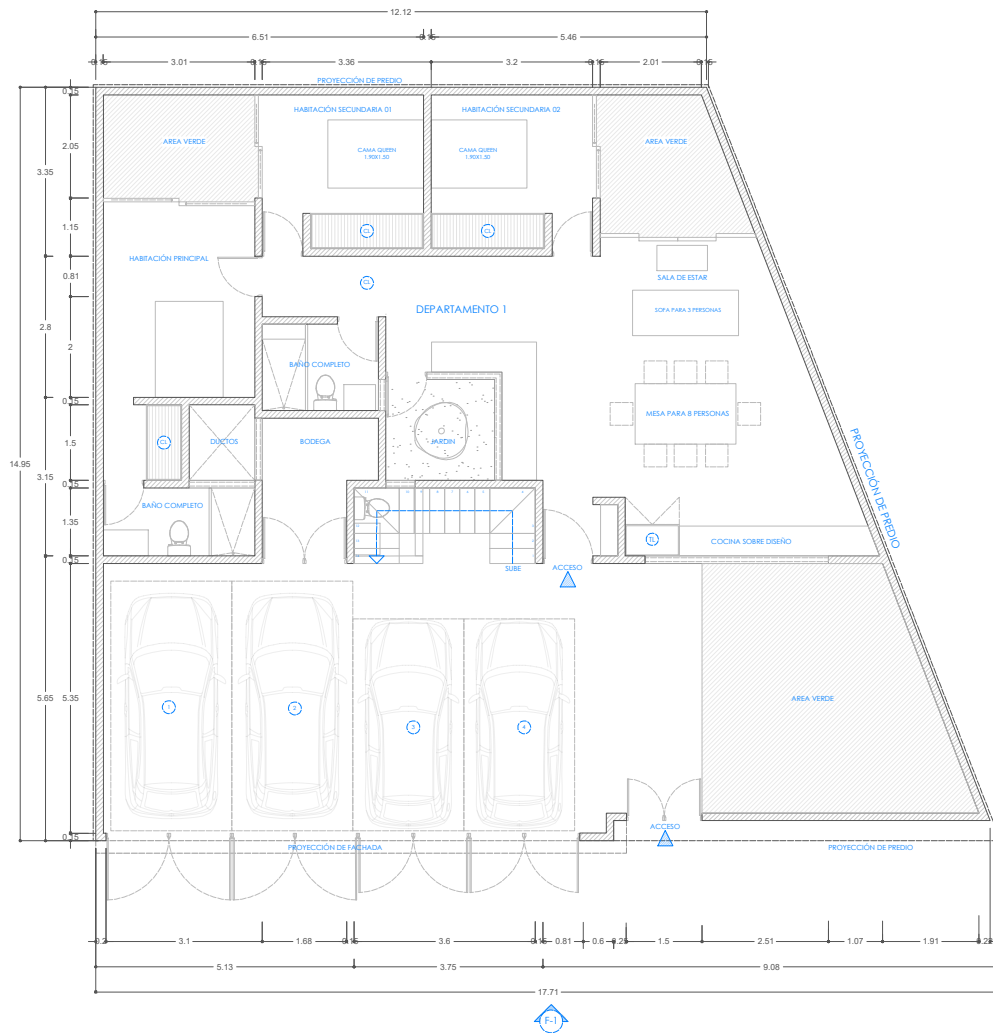
PLANTA BAJA
